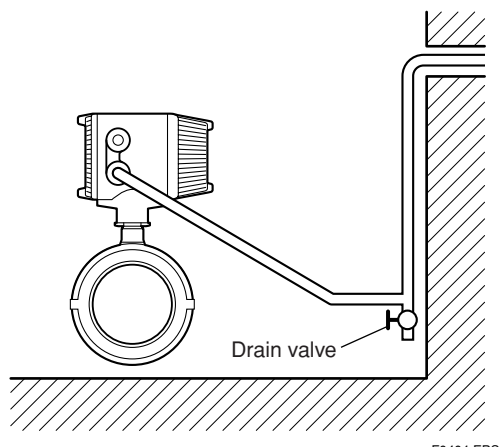
Figure 4.1.4 Conduit Wiring
